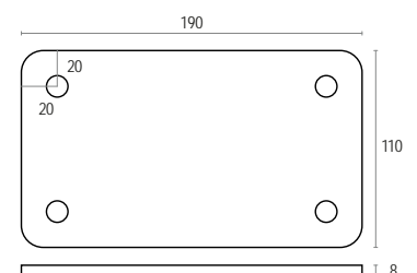
Piastra tassellare per recinzioni H 1600 - 1800 - 2000
