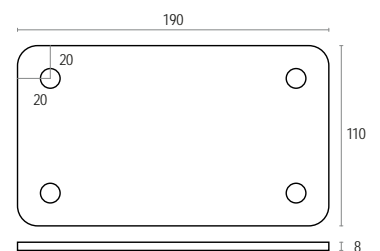
Piastra tassellare per recinzioni H 1600 - 1800 - 2000
