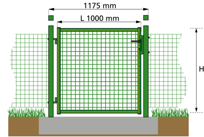
CANCELLETTO 1 ANTA Colonne da annegare \varnothing 50/60 mm telaio \varnothing 35/40 mm specchiatura in rete elettrosaldata con toni \varnothing 4 mm larghezza anta 1000 mm zincato a caldo e plastificato.
