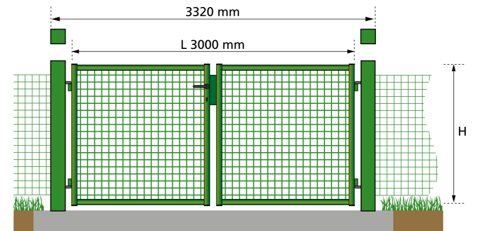
CANCELLO 2 ANTE Colonne da annegare \varnothing 100 mm telaio \varnothing 35/40 mm specchiatura in rete elettrosaldata con toni \varnothing 4 mm larghezza anta 1500 mm zincato a caldo e plastificato.
