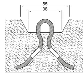
Guida incassata nel pavimento
