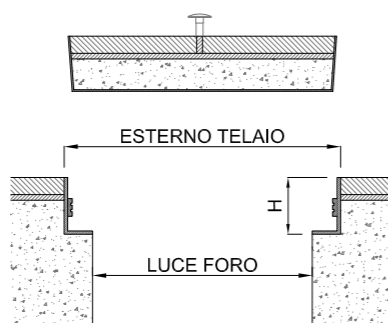
I chiusini Lock sono provvisti di guarnizione perimetrale sul telaio.
