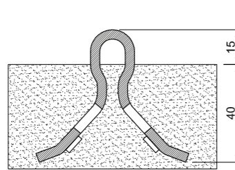
Guida sporgente dal pavimento
