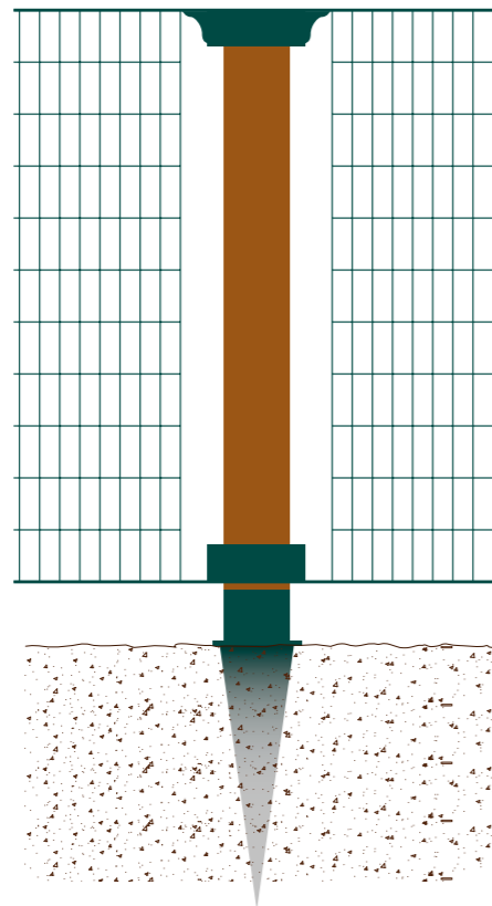
Fissaggio Ring® e base ad annegare
