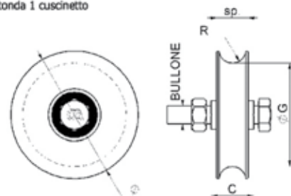
Ruota gola tonda 1 cuscinetto
