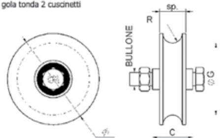
Ruota gola tonda 2 cuscinetti
