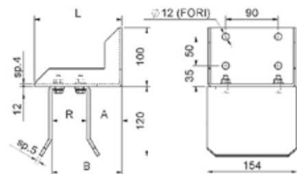
Incontro superiore universale regolabile zincato
