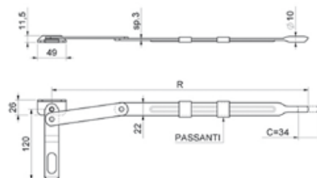
PALETTO A LEVA ZINCATO con passanti di guida
