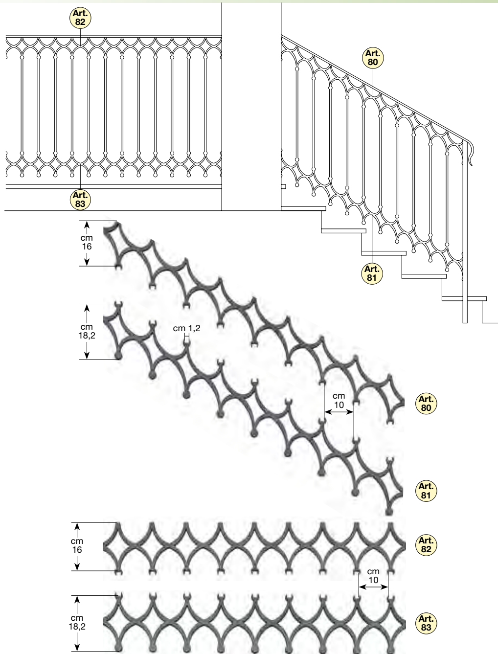
Art. 80 - 81 - 82 - 83 da cm 100 - 150 - 200 spessore mm 10.
