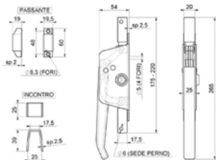
Cariglione quadro 14 zincato c/cilindro
