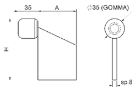
Arresto fine corsa zincato
