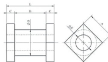
Tronchetto di giunzione per cardine a fascetta
