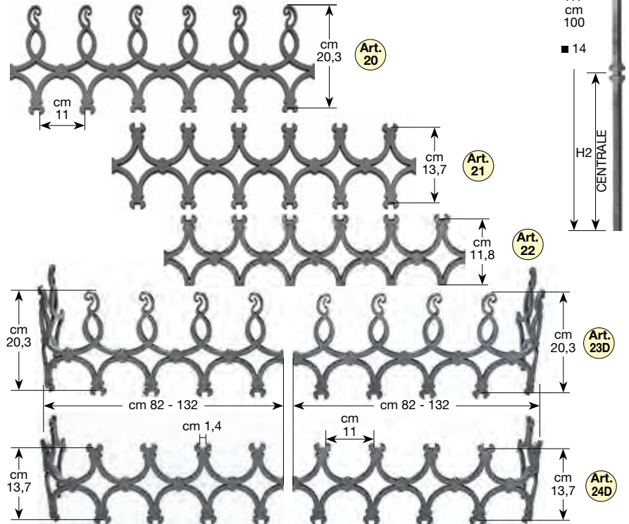
Art. 20 - 21 - 22 da cm 100 - 150 - 200 spessore mm 10. Art. 23D - 23S - 24D - 24S - da cm 100 - 150 spessore mm 10. Vengono forniti piegati su un lato.
