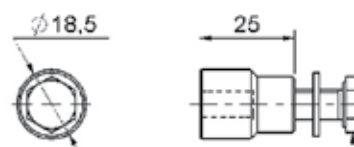
VITE TE M8x25 CON RONDELLA
