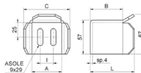
Incontro superiore zincato regolabile
