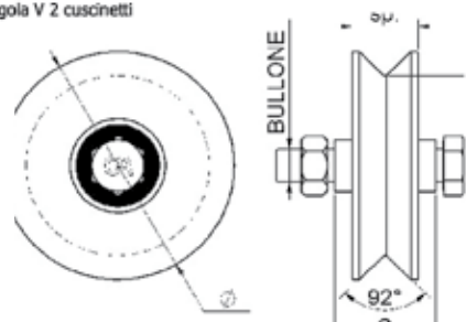
Ruota gola V 2 cuscinetti
