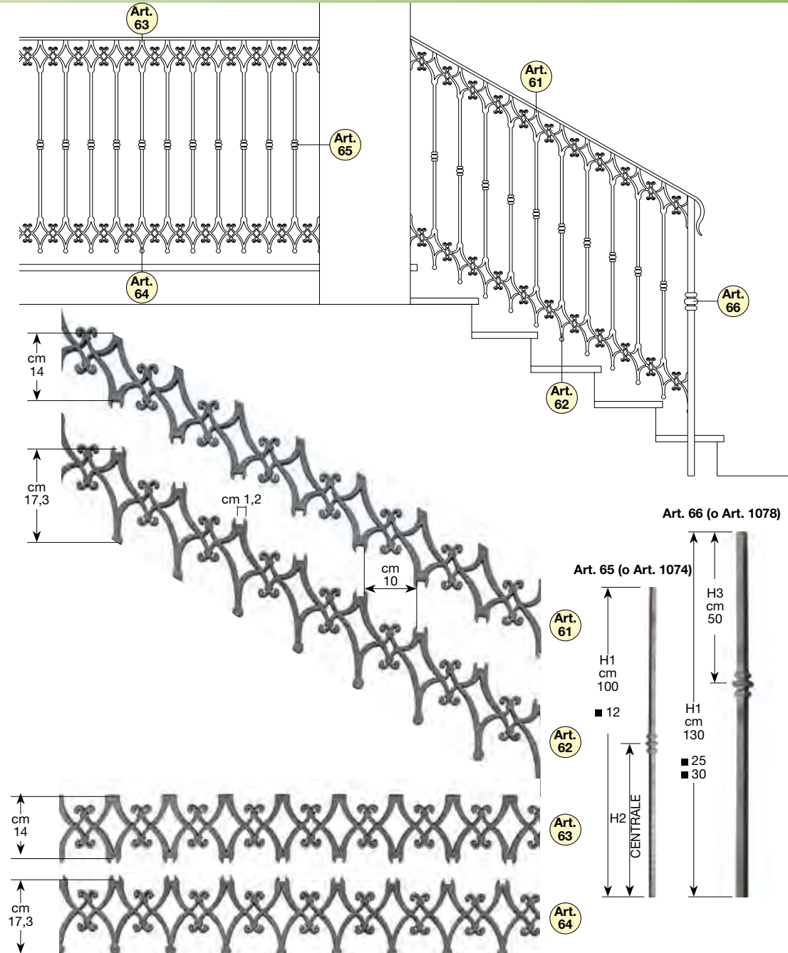
Art. 61 - 62 - 63 - 64 da cm 100 - 150 - 200 spessore mm 10.
