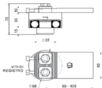
Cardine regolabile zincato c/cuscinetto
