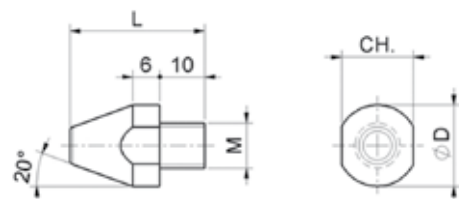
Antistrappo perno filettato
