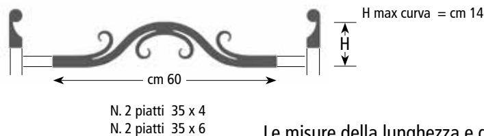
Art. BL 254 Si forniscono solo lisce
