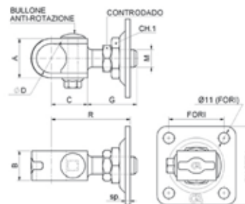
Cardine a fascetta regolabile c/piastra Zincato
