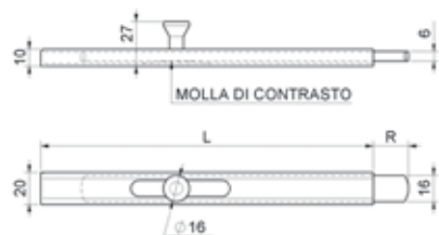
Catenaccio verticale zincato
