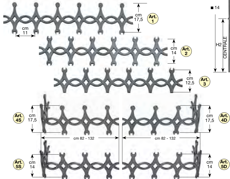
Art. 1 - 2 - 3 da cm 100 - 150 - 200 spessore mm 10. Art. 4S - 4D - 5S - 5D - da cm 100 - 150 spessore mm 10. Vengono forniti piegati su un lato.
