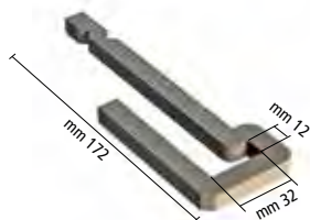
Supporto di fissaggio per inferriata sporgente in lamiera.
