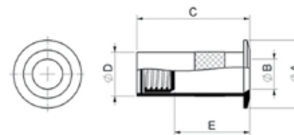
Pozzetto in ottone antipolvere c/molla inox
