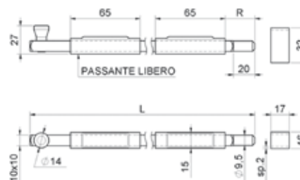
Catenaccio verticale 10x10 zincato c/punta tonda
