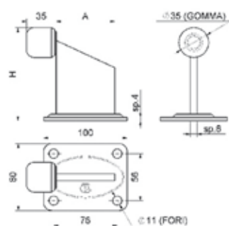
Arresto fine corsa zincato c/piastra a fissare
