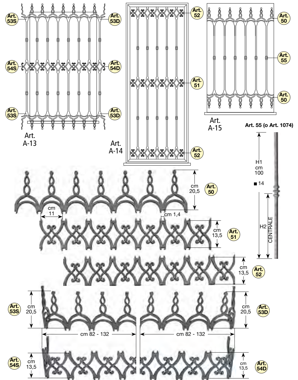
Art. 50 - 51 - 52 da cm 100 - 150 - 200 spessore mm 10. Art. 53D - 53S - 54D - 54S - da cm 100 - 150 spessore mm 10. Vengono forniti piegati su un lato.
