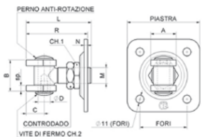
Cardine con alette c/piastra Zincato
