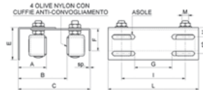
Piastra guida regolabile 4 olive nylon
