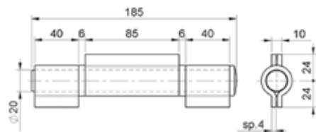
Cerniera per cancelli 3 all corte con perno zincato e rondelle ottone
