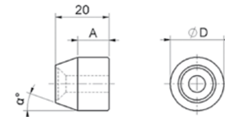
Antistrappo per vite testa svasata
