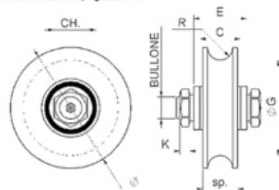
Ruota gola tonda 2 cuscinetti c/ingrassatore
