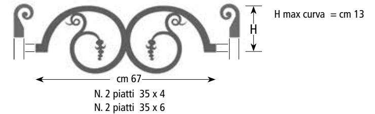
Art. BL 256 Si forniscono solo lisce
