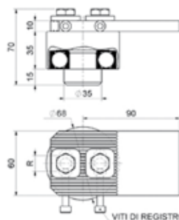
CARDINE CON CUSCINETTO ZINCATO - REGOLABILE
