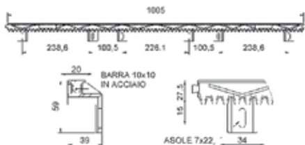
Cremagliera nylon c/attacchi inferiori - mod. medio
