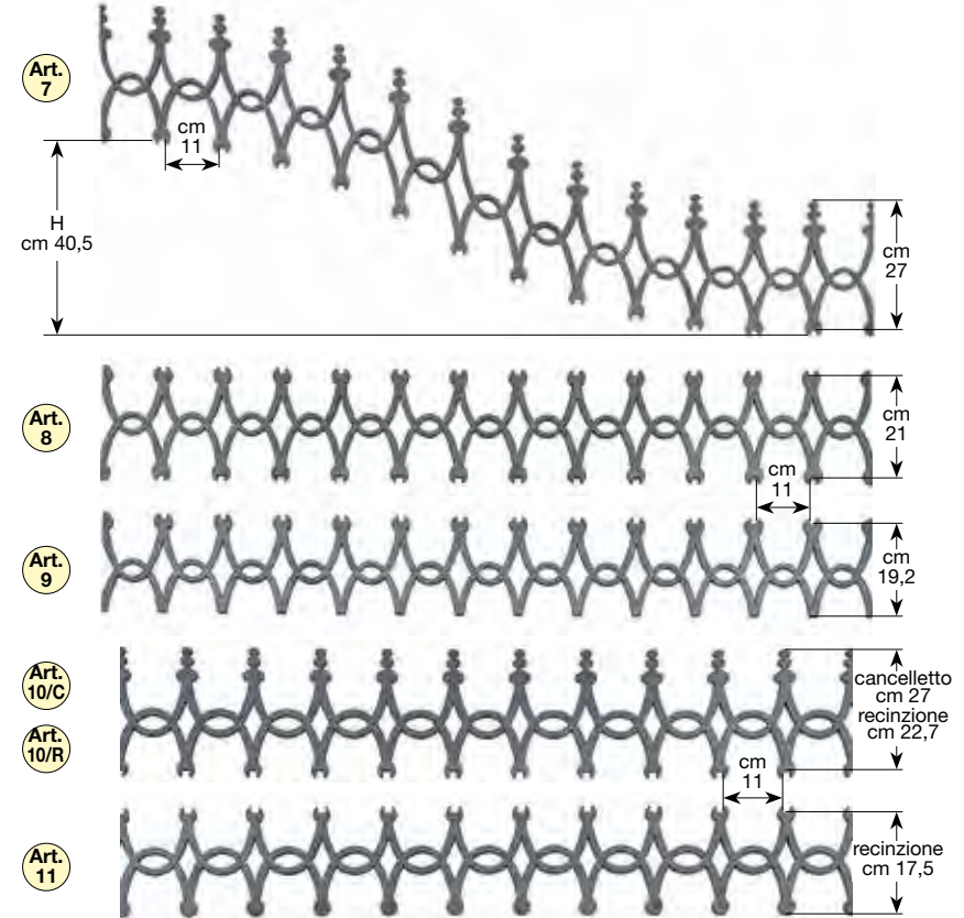
Art. 7 da cm 200 - 250 spessore mm 10. Art. 8 - 9 da cm 100 - 150 - 200 - 250 spessore mm 10. Art. 10 - 11 da cm 100 - 150 - 200 spessore mm 10.
