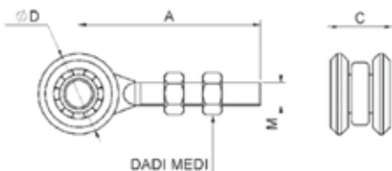
Carrello scorrevole zincato 2 ruote/cuscinetti
