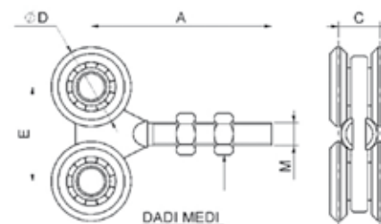
Carrello scorrevole zincato 4 ruote/cuscinetti
