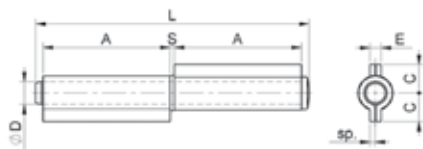
Cerniera 2 all perno sfilabile
