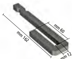
Supporto di fissaggio per inferriata interna in lamiera.
