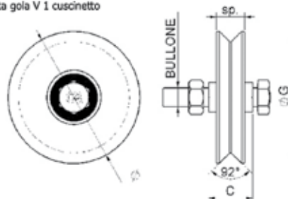
Ruota gola V 1 cuscinetto
