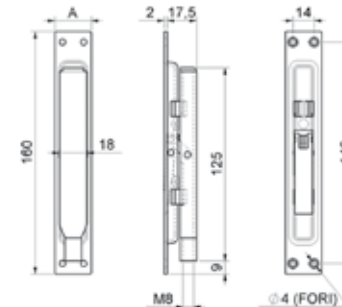
Catenaccio UNA azione c/leva OTTONE Zincato
