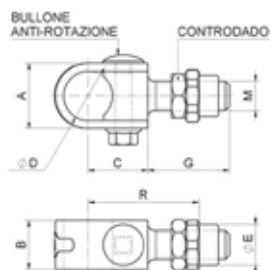
Cardine a fascetta c/boccola Zincato
