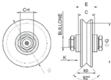
Ruota gola V 1 cuscinetto c/ingrassatore
