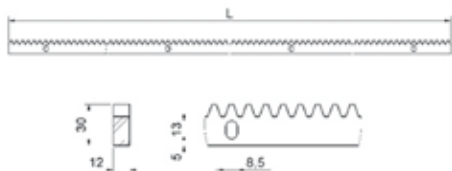
Cremagliera zincata rettangolare 30x12 m.4
