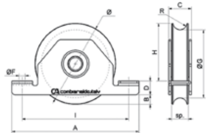
Ruota gola tonda 1 cuscinetto supporto interno
