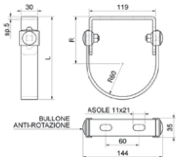
Anello di sicurezza zincato
