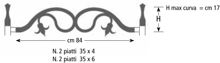
Art. BL 252 Si forniscono solo lisce
