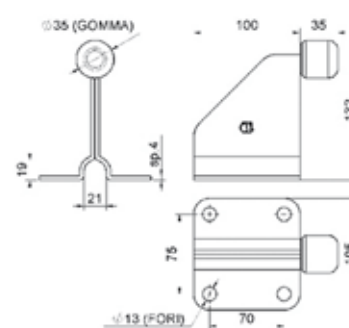
Arresto fine corsa con piastra copri-binario a fissare Zincato
