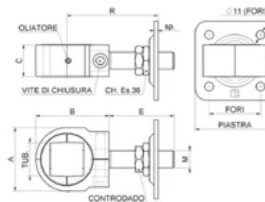
Cardine MATRIX c/piastra con ingrass. Zincato
