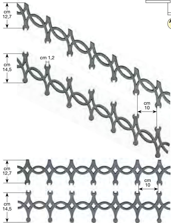
Art. 12 - 13 - 14 - 15 da cm 100 - 150 - 200 spessore mm 10.
