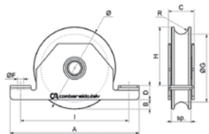
Ruota gola tonda 2 cuscinetti supporto interno
