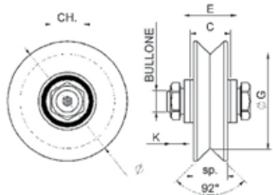
Ruota gola V 2 cuscinetti c/Ingrassatore
