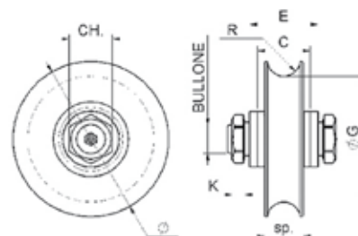
Ruota gola tonda 1 cuscinetto c/ingrassatore
