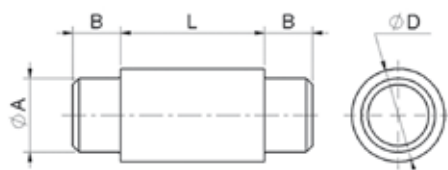
Tronchetto di giunzione tondo per cardine a fascetta
