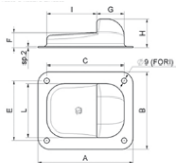
Battente d'arresto a fissare Zincato
