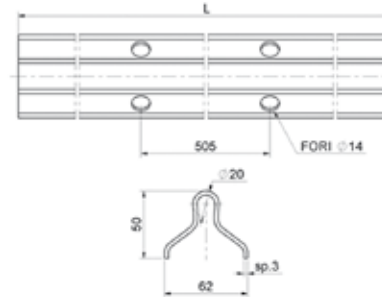
Binario Tondo Aperto Ø20 a cementare Zincato
