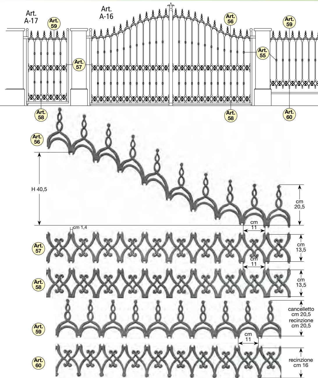
Art. 56 da cm 200 - 250 spessore mm 10. Art. 57 - 58 da cm 100 - 150 - 200 - 250 spessore mm 10. Art. 59 - 60 da cm 100 - 150 - 200 spessore mm 10.
