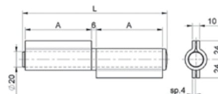
Cerniera per cancelli 2 all corte perno zincato e rondella ottone
