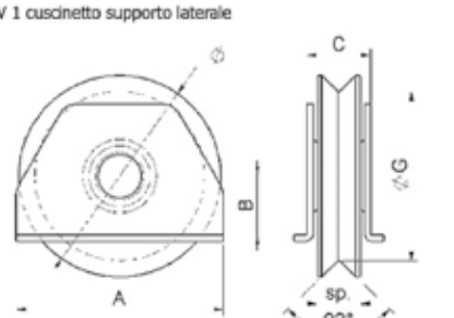
Ruota gola V 1 cuscinetto supporto laterale
