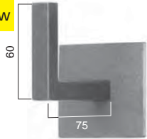
Piastra/Plate H.60 X 60 mm. ≠ 5 mm. Art. 15.005.10 □ 12 mm.
