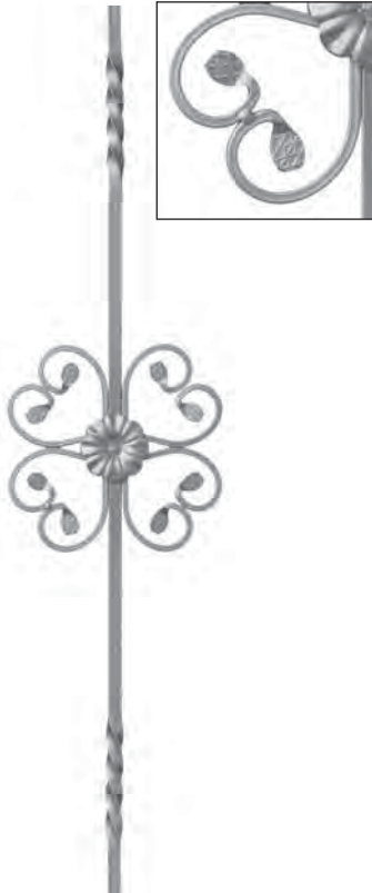
🌀 Liscio / Smooth H. 950 X L. 190 mm. Art. 05.800 □ 12 ≠ 12 x 6
