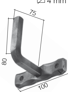
Art. 1405/1 Base 25 x 8 mm holes-foi Ø 8,5 mm ∩ 12 x 12 mm
