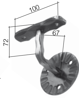
Art. 1405/2 Base Ø 80 x 4 mm holes-foi Ø 8,5 mm ∩ 12 x 12 mm
