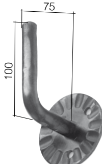
Art. 1405/3 Base Ø 80 x 4 mm holes-foi Ø 8,5 mm Ø 16 mm
