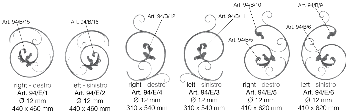
right - destro Art. 94/C/9 Ø 12 mm 280 x 390 mm left - sinistro Art. 94/C/10 Ø 12 mm 280 x 390 mm right - destro Art. 94/C/11 Ø 12 mm 330 x 370 mm left - sinistro Art. 94/C/12 Ø 12 mm 330 x 370 mm right - destro Art. 94/C/13 Ø 12 mm 330 x 510 mm left - sinistro Art. 94/C/14 Ø 12 mm 330 x 510 mm
