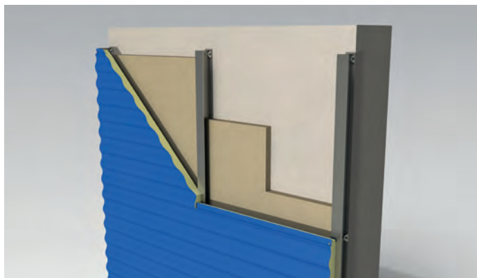
A lato: schema di facciata ventilata realizzata su parete esistente e pannello ONDA. On the side: scheme of ventilated facade built on existing wall and ONDA panel.
